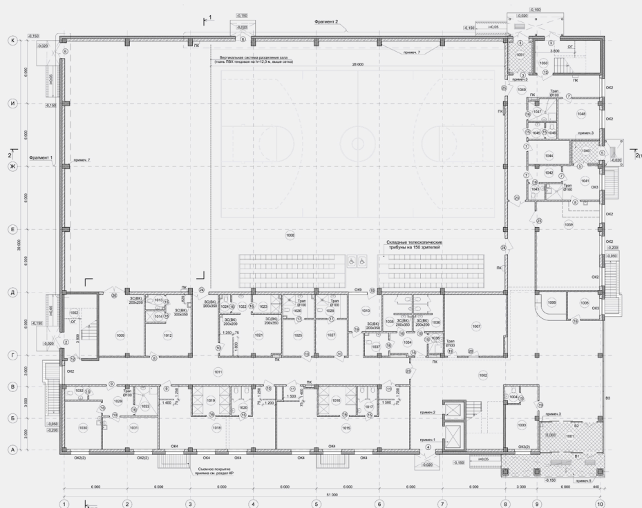
ПЛАН 2 ЭТАЖА
