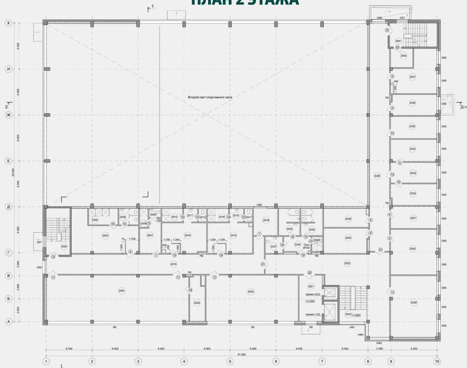
ПЛАН 2 ЭТАЖА
